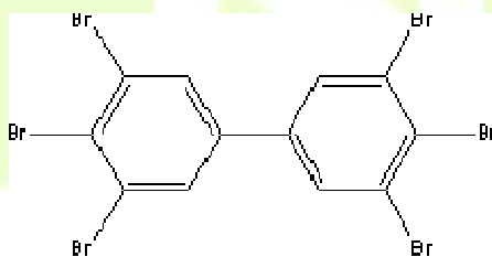
Obrázek 1: Struktura hexabrombifenylu
