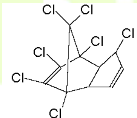
Obrázek 1: Molekula heptachloru
