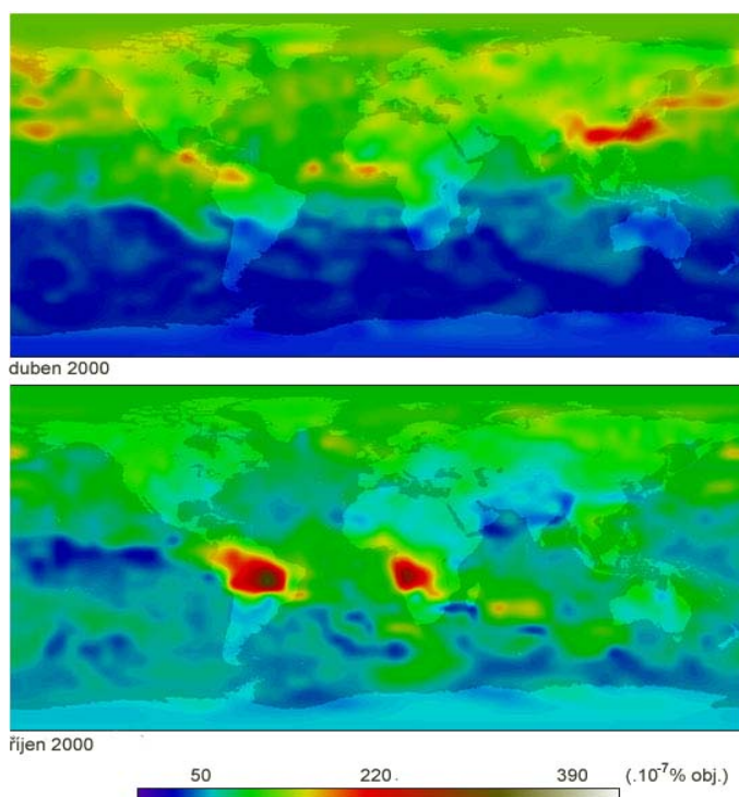
Obr. 1. Satelitní snímek Země s obsahy oxidu uhelnatého ve spodních vrstvách atmosféry pořízený geografickým satelitem NASA „Terra“ s pomocí senzoru „MOPITT“.
